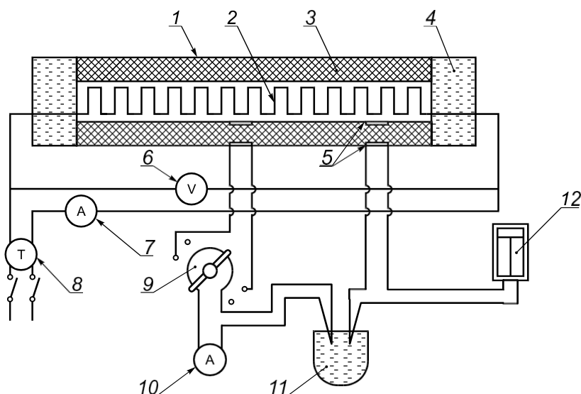
1 — стальная труба; 2 — электронагреватель; 3 — испытуемый материал; 4 — охранный секция; 5 — термодатчики; 6 — вольтметр; 7 — амперметр; 8 — автотрансформатор; 9 — переключатель; 10 — гальванометр; 11 — сосуд со льдом; 12 — самопишущий гальванометр
